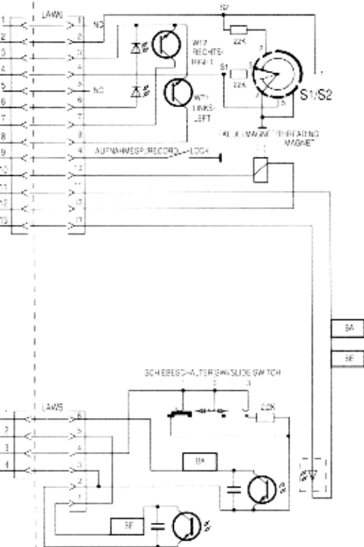
Chassisplatte - Ablaufsteuerung Chassis Board - Sequence Control
